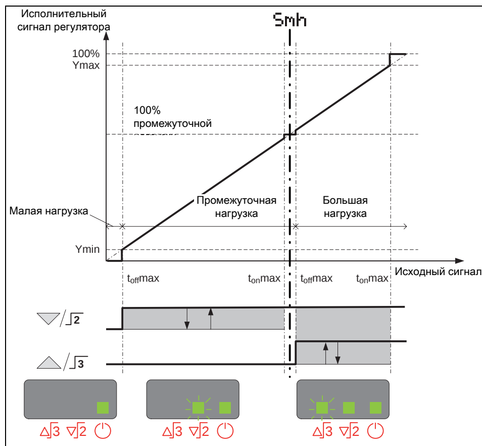
Рис. 14: Переключающийся регулятор
