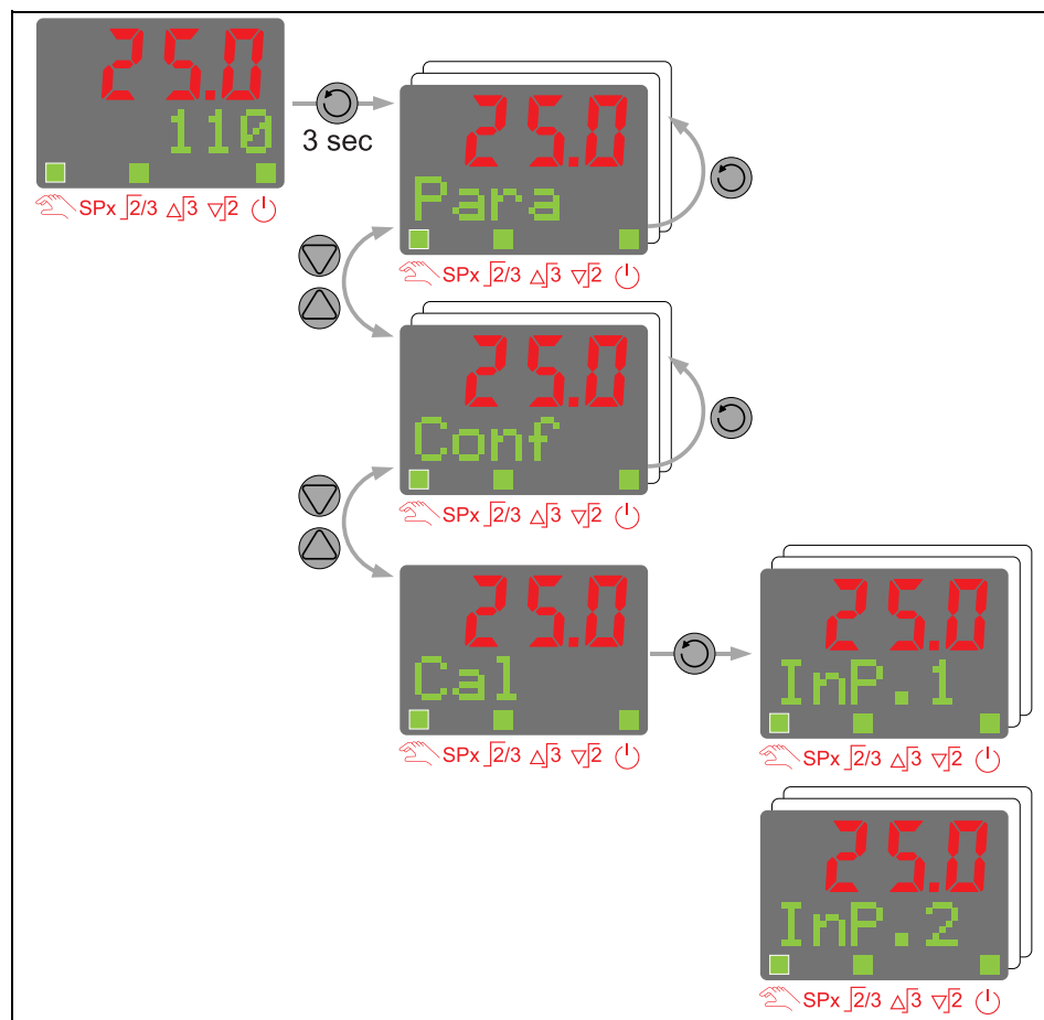
Рис. 15: Уровень калибровки
