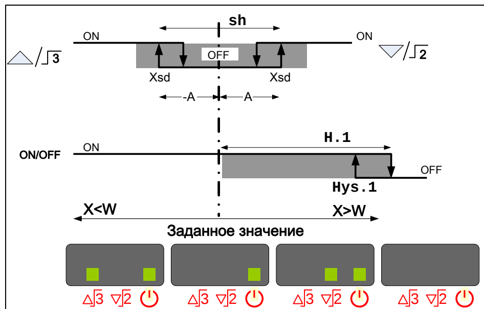
Рис. 13: 3-точечный регулятор
