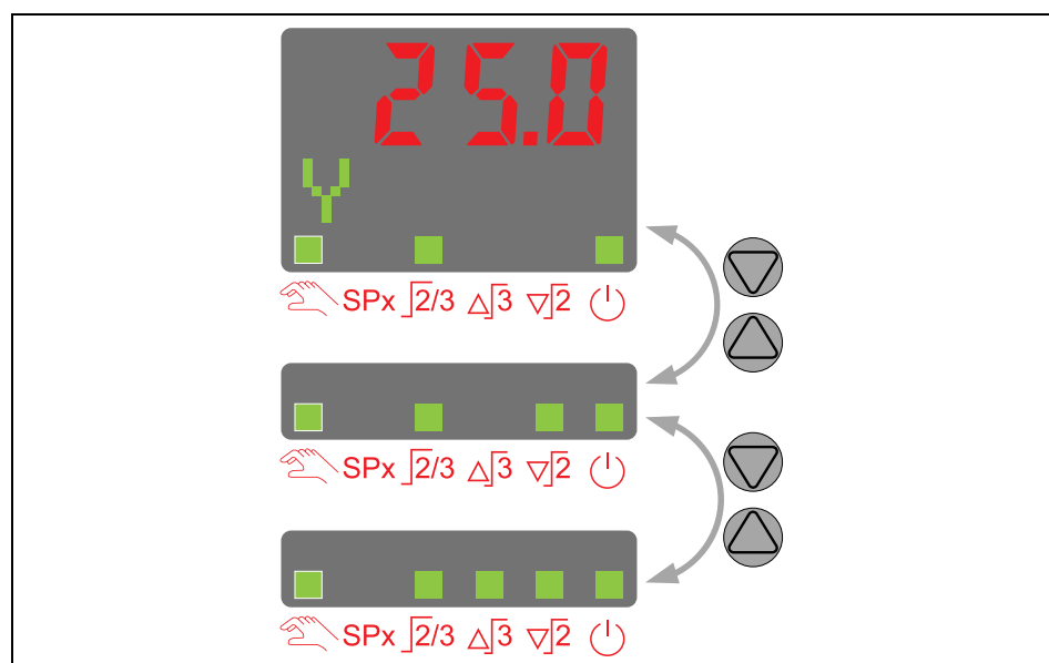
Рис. 9: Ступенчатый регулятор
