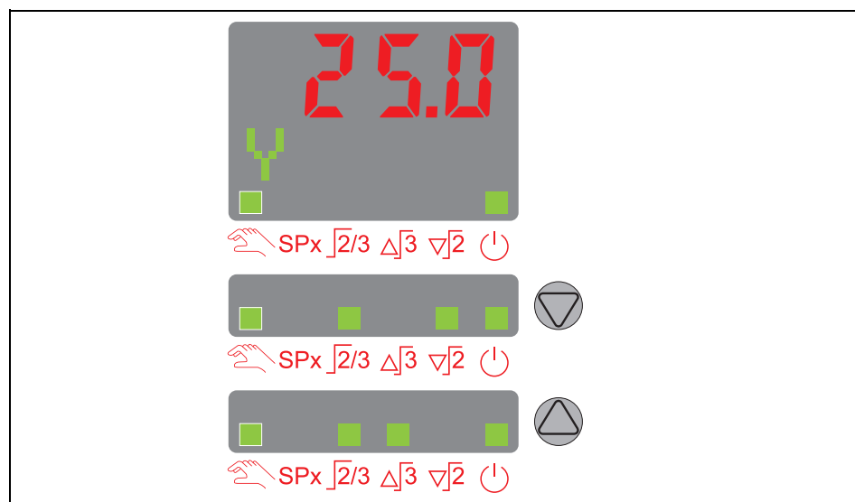
Рис. 8: 3-точечный регулятор
