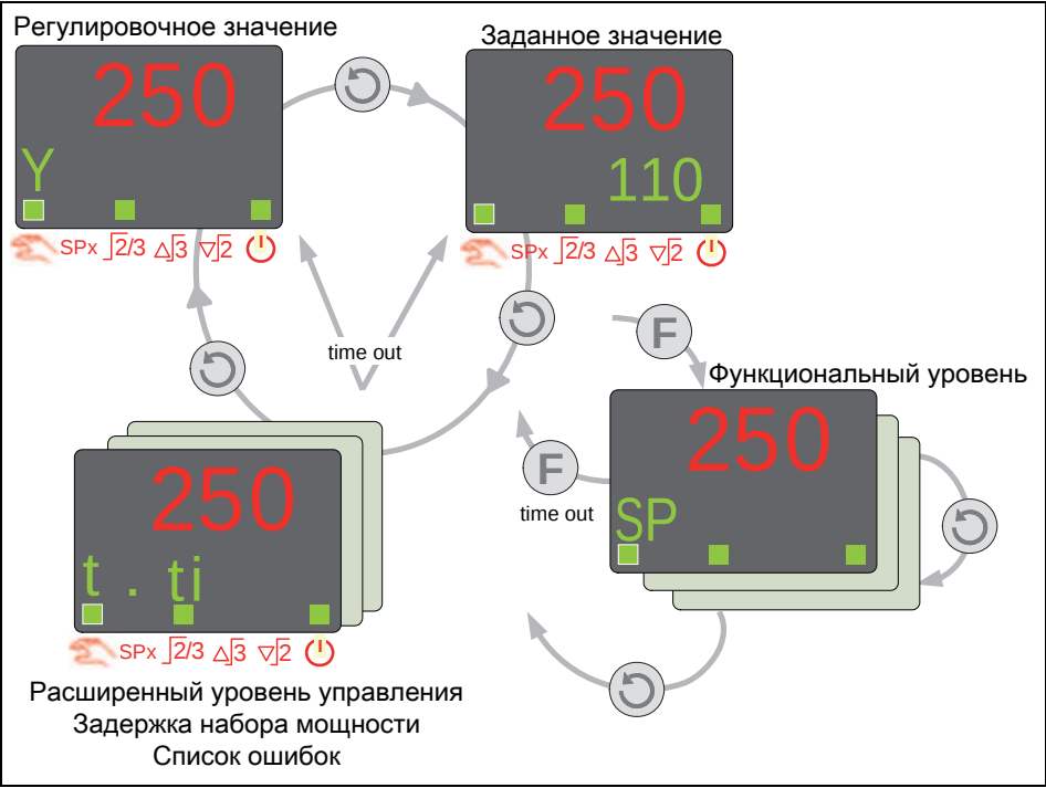
Рис. 6: Уровень управления
